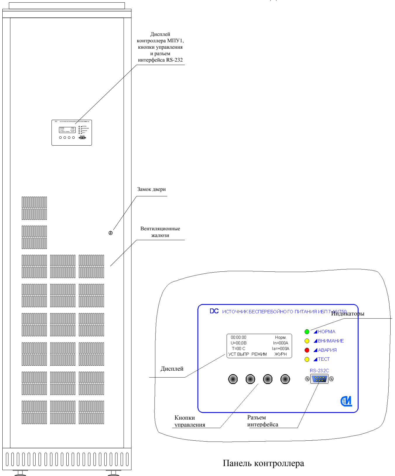
Рис.3.2 Общий вид устройства ИБП7-48/900-18.N-КТА с закрытой передней дверью. Общий вид панели контроллера.
