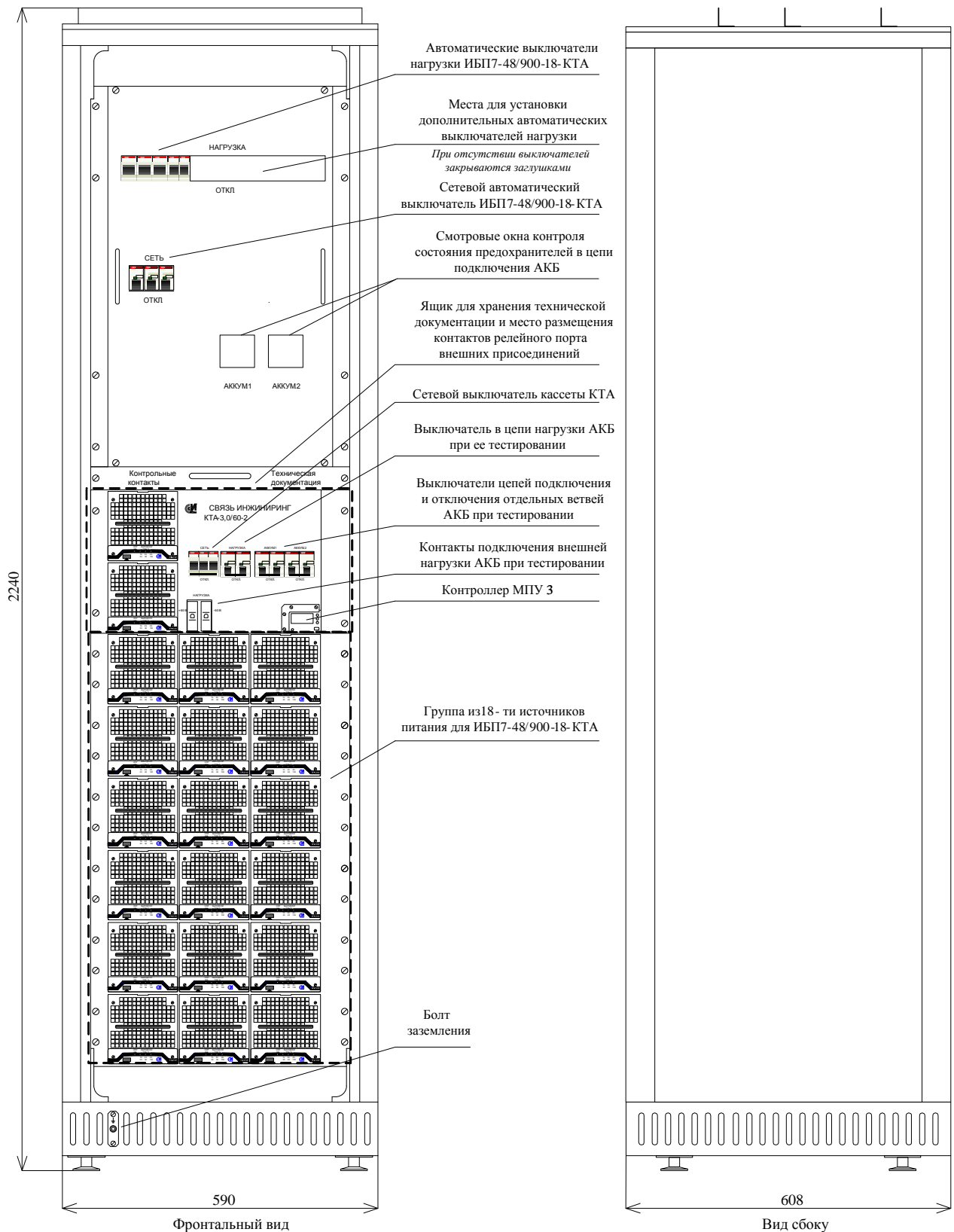
Рис.3.1 Общий вид и габаритные размеры устройства ИБП7-48/900-18.N-КТА с 18 блоками питания и кассетой КТА.
