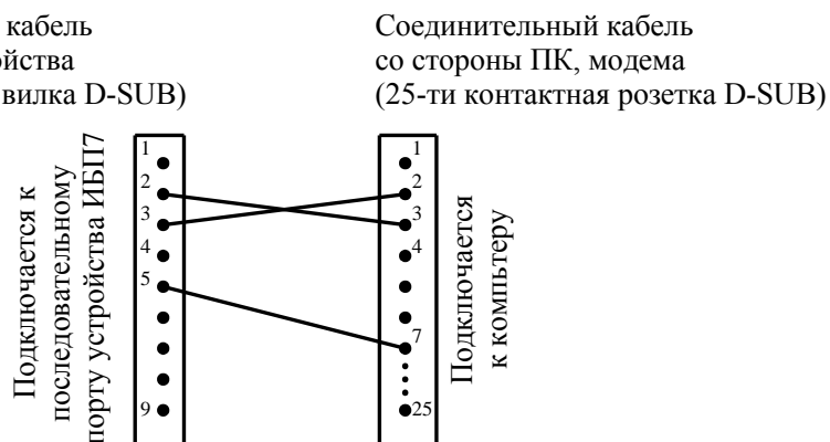
Рис.3.3б Схема распайки соединительного кабеля типа 2 – для ПК, модема с 25-контактным разъемом последовательного порта
