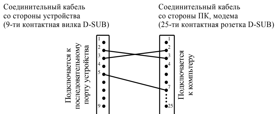
Рис.3.3б Схема распайки соединительного кабеля типа 2 – для ПК, модема с 25-контактным разъемом последовательного порта
