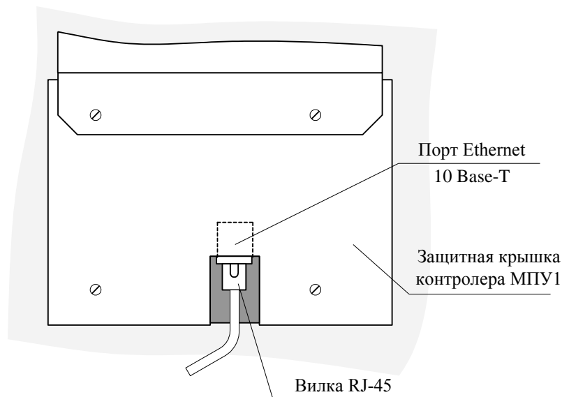
Рис.3.3 Расположение разъема порта Ethernet
