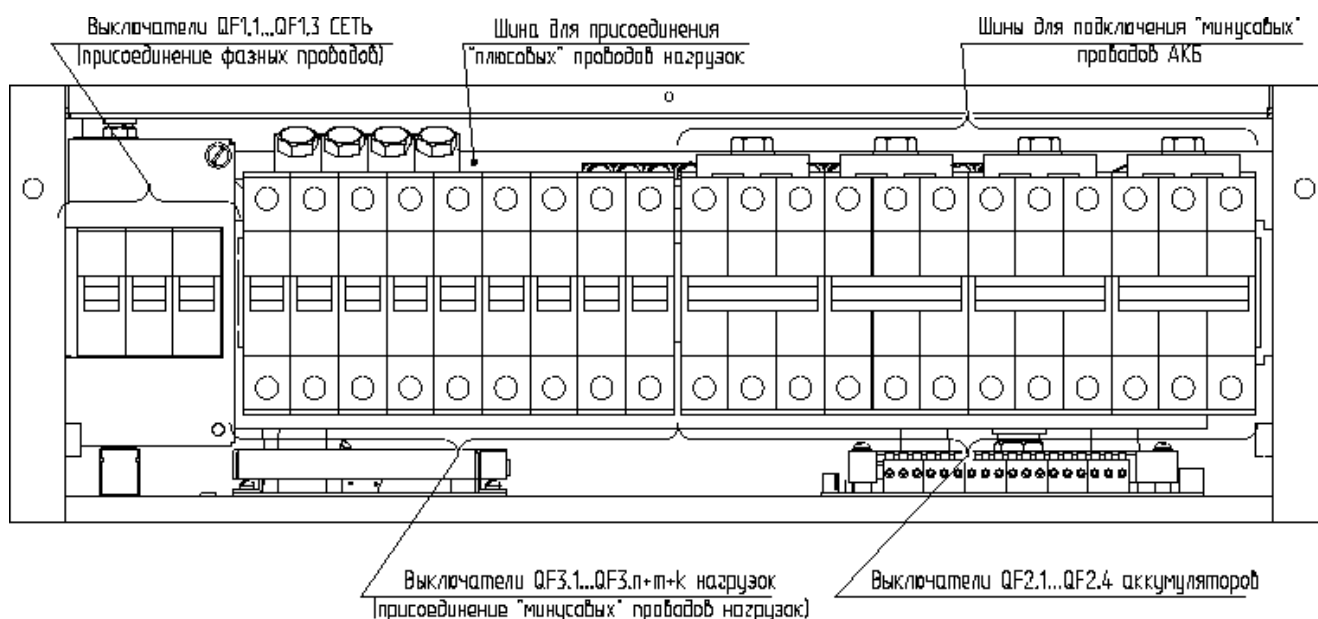
Рис.3.4 Общий вид элементов внешних подключений (модуль управления с открытой передней панелью).
