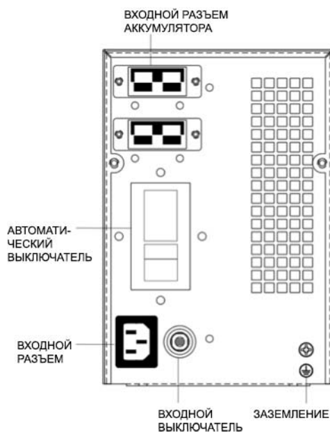
Рисунок 2 Задняя панель аккумуляторного блока 1 кВА
