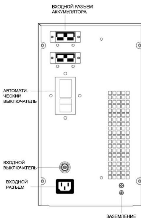
Рисунок 3 Задняя панель аккумуляторного блока 1,5 кВА/ 2кВА/ 3 кВА
